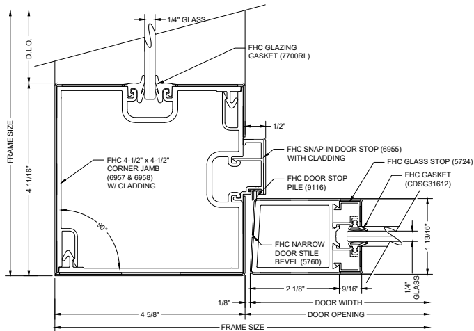
G4 90° CORNER DOOR JAMB
