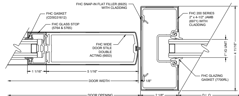
E26 DOOR & SIDELITE JAMB
