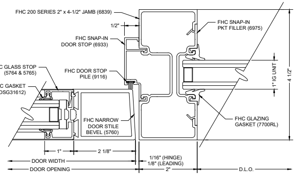
E7 DOOR & SIDELITE JAMB
