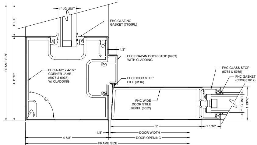
G12 90° CORNER DOOR JAMB
