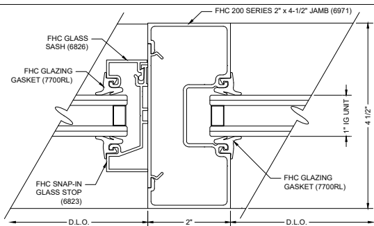
Q7 JAMB @ TRANSOM
