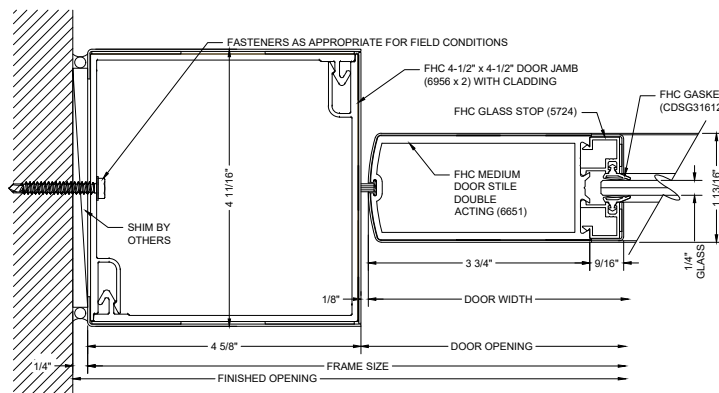
G31 DOOR JAMB @ WALL
