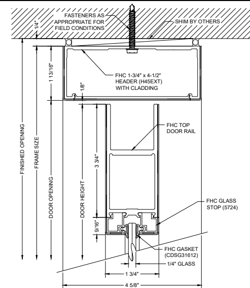
B7 DOOR HEADER
