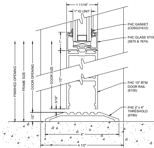
C8 BOTTOM OF DOOR
