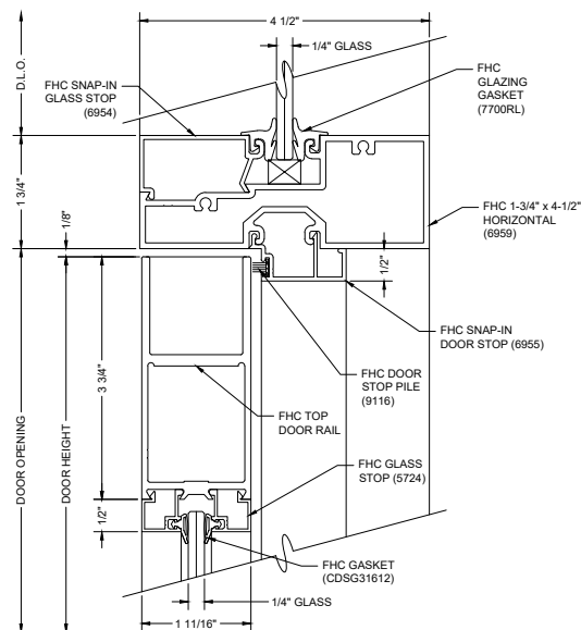
A1 DOOR & TRANSOM HEADER
