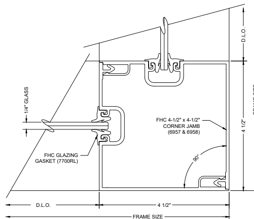
N1 90° CORNER JAMB
