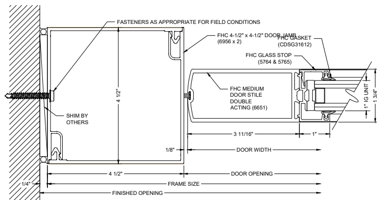
G34 DOOR JAMB @ WALL
