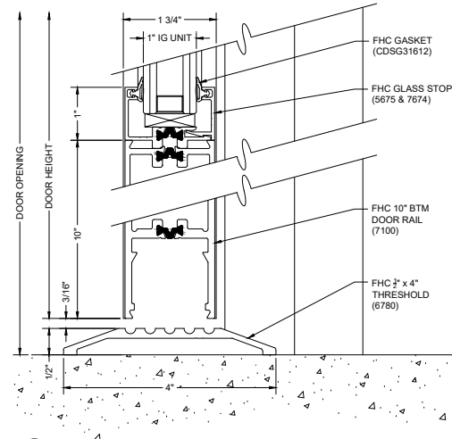
C5 BOTTOM OF DOOR
