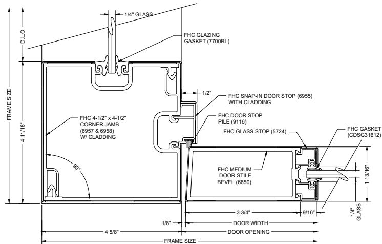
G5 90° CORNER DOOR JAMB
