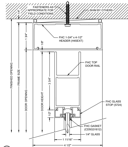
B6 DOOR HEADER
