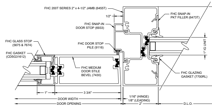
E13 DOOR & SIDELITE JAMB
