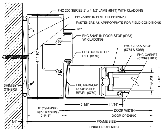
F10 DOOR JAMB @ WALL
