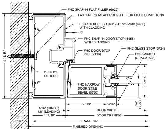
F4 DOOR JAMB @ WALL
