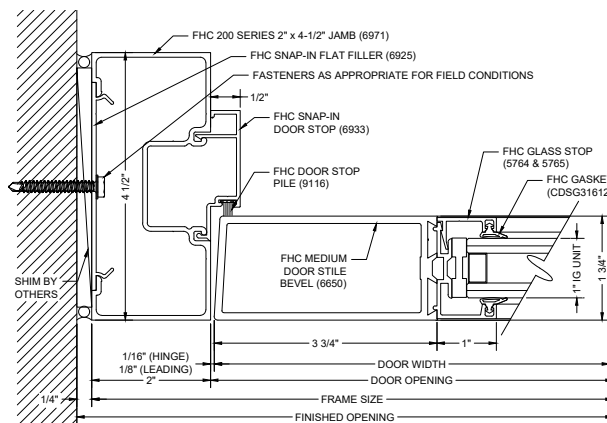
F8 DOOR JAMB @ WALL
