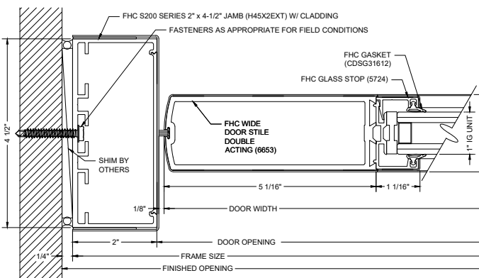
F26 DOOR JAMB @ WALL
