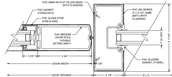
E25 DOOR & SIDELITE JAMB
