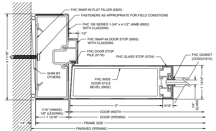
F6 DOOR JAMB @ WALL
