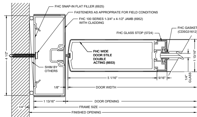
F20 DOOR JAMB @ WALL
