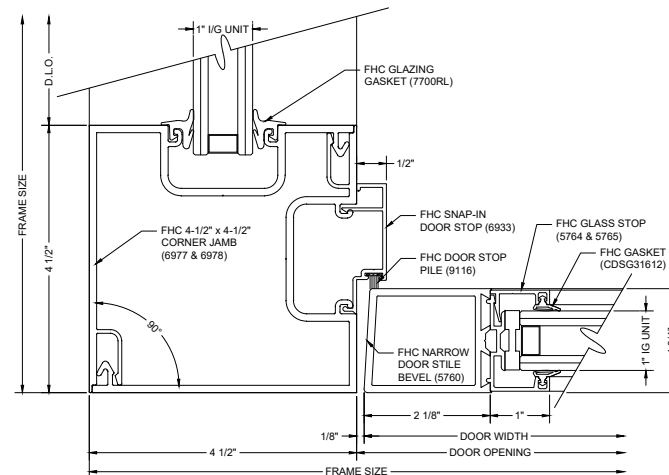
G7 90° CORNER DOOR JAMB
