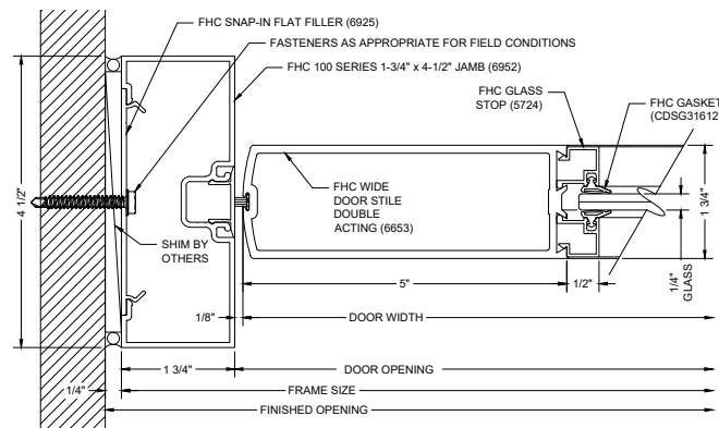
F17 DOOR JAMB @ WALL
