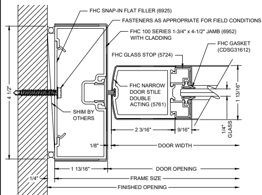
F18 DOOR JAMB @ WALL
