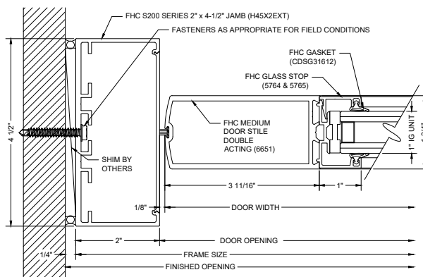
F22 DOOR JAMB @ WALL
