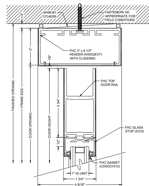
B9 DOOR HEADER
