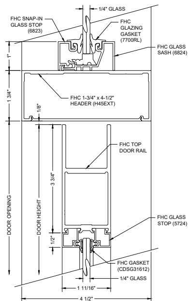
A6 DOOR & TRANSOM HEADER
