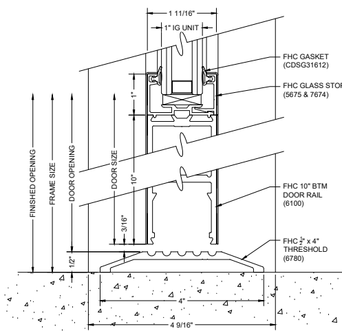
C9 BOTTOM OF DOOR
