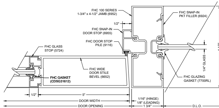
E3 DOOR & SIDELITE JAMB
