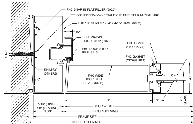
F3 DOOR JAMB @ WALL
