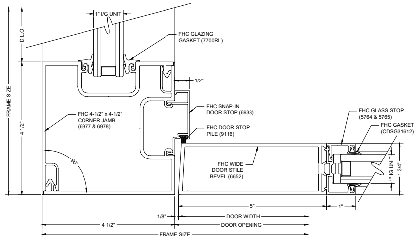
G9 90° CORNER DOOR JAMB
