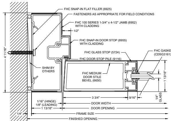
F5 DOOR JAMB @ WALL
