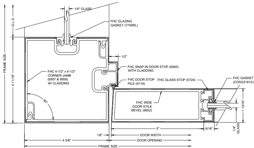
G6 90° CORNER DOOR JAMB
