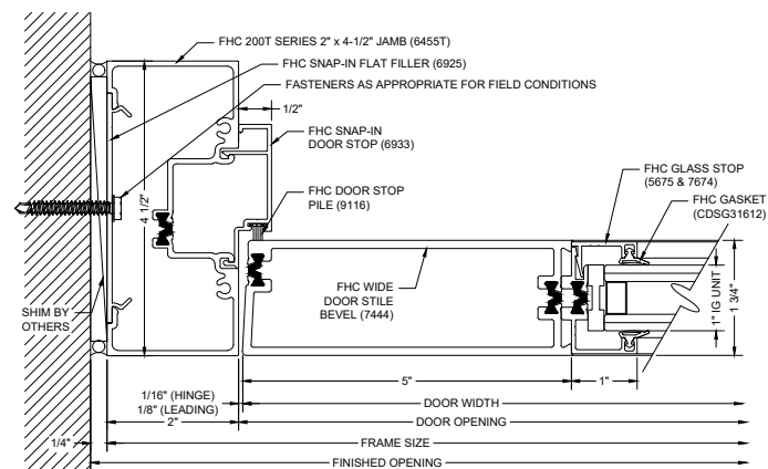
F14 DOOR JAMB @ WALL
