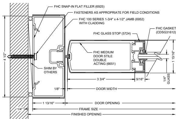
F19 DOOR JAMB @ WALL
