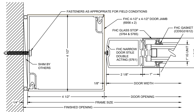
G33 DOOR JAMB @ WALL
