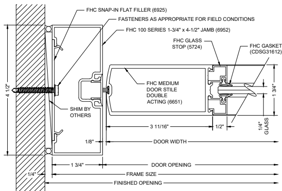
F16 DOOR JAMB @ WALL
