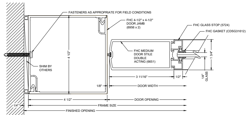
G28 DOOR JAMB @ WALL
