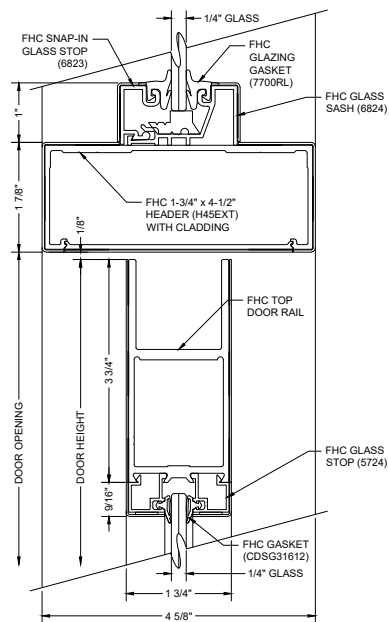
A7 DOOR & TRANSOM HEADER
