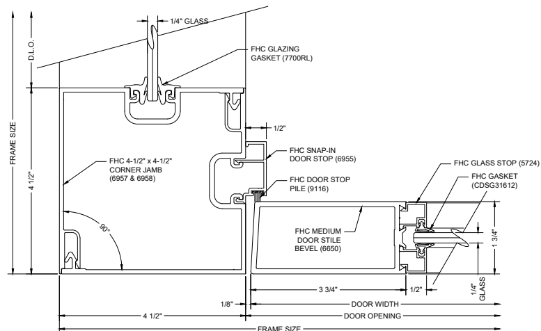
G2 90° CORNER DOOR JAMB
