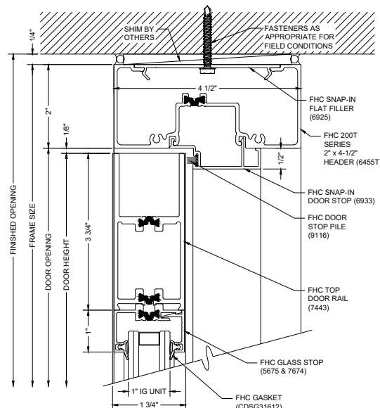
B5 DOOR HEADER
