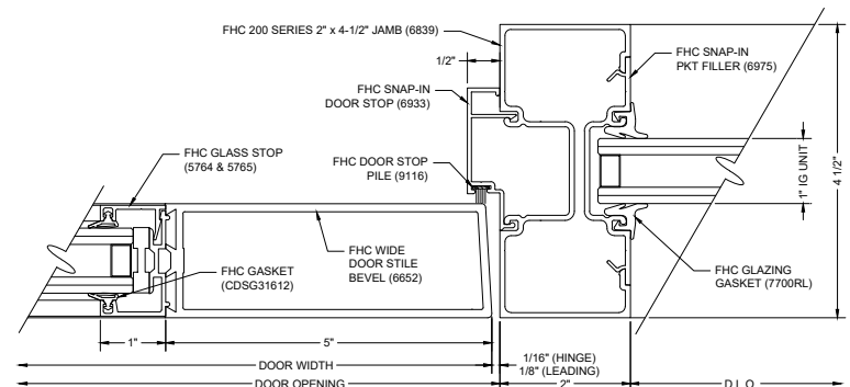
E9 DOOR & SIDELITE JAMB
