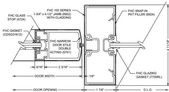
E18 DOOR & SIDELITE JAMB
