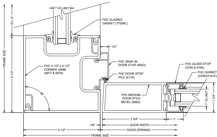
G8 90° CORNER DOOR JAMB
