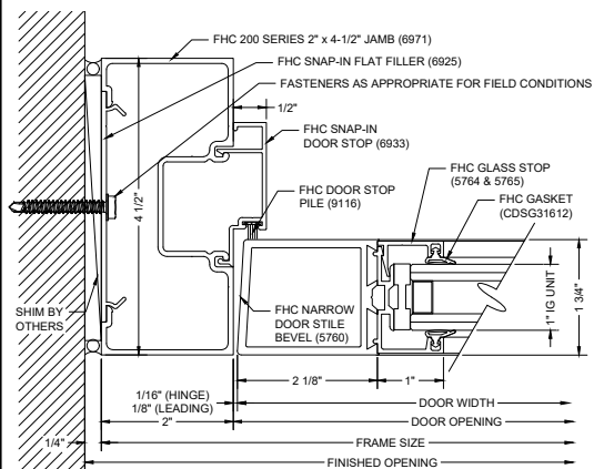
F7 DOOR JAMB @ WALL
