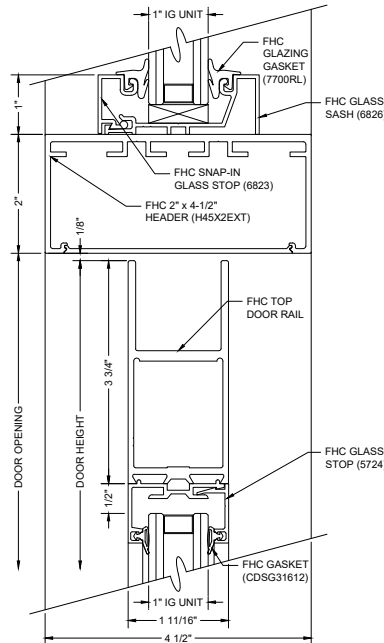
A8 DOOR & TRANSOM HEADER
