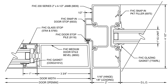
E8 DOOR & SIDELITE JAMB
