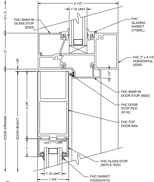
A3 DOOR & TRANSOM HEADER
