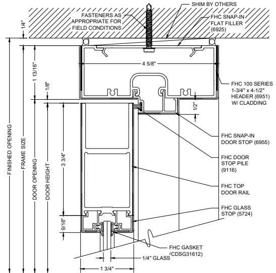
B2 DOOR HEADER
