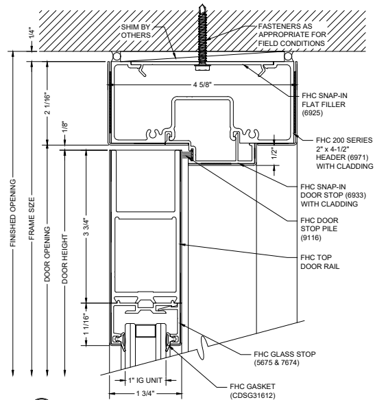
B4 DOOR HEADER
