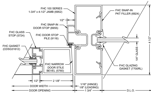
E1 DOOR & SIDELITE JAMB
