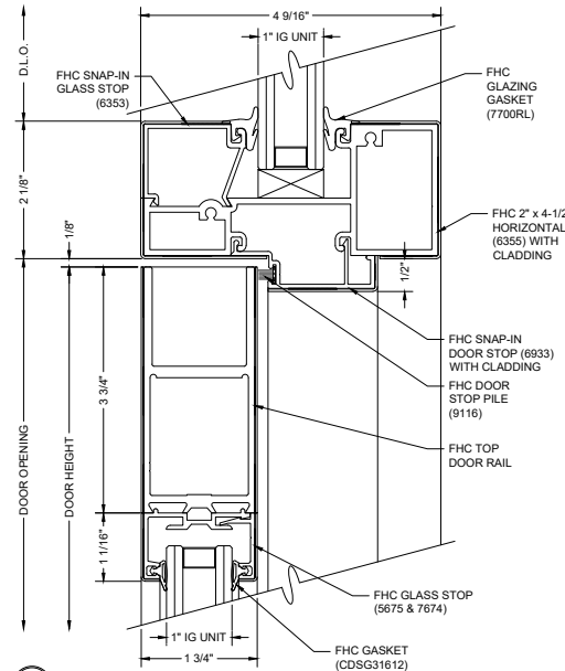
A4 DOOR & TRANSOM HEADER
