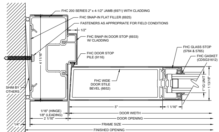
F12 DOOR JAMB @ WALL
