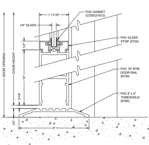
C1 BOTTOM OF DOOR
