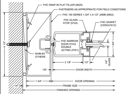
F15 DOOR JAMB @ WALL
