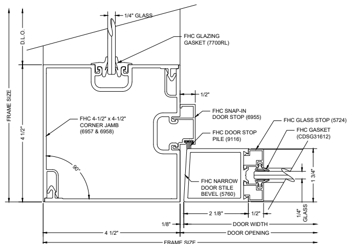
G1 90° CORNER DOOR JAMB
