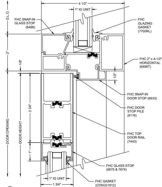
A5 DOOR & TRANSOM HEADER
