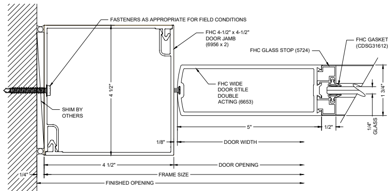
G29 DOOR JAMB @ WALL
