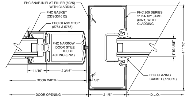
E24 DOOR & SIDELITE JAMB
