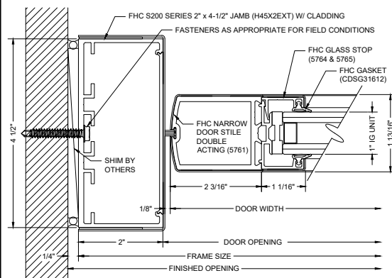
F24 DOOR JAMB @ WALL
