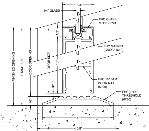
C7 BOTTOM OF DOOR
