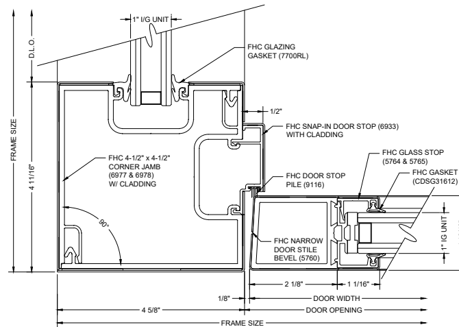
G10 90° CORNER DOOR JAMB
