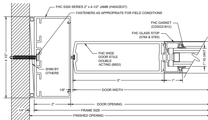
F23 DOOR JAMB @ WALL
