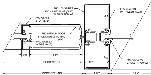
E19 DOOR & SIDELITE JAMB
