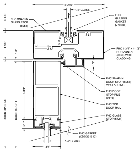
A2 DOOR & TRANSOM HEADER
