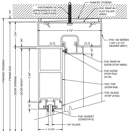
B1 DOOR HEADER
