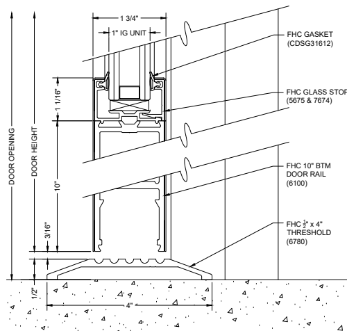
C4 BOTTOM OF DOOR
