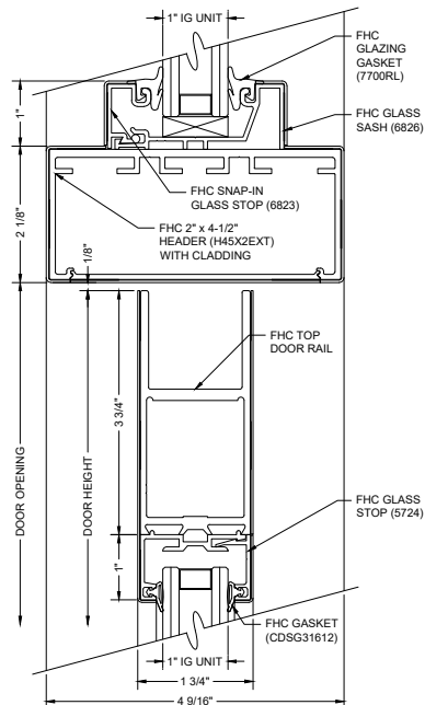
A9 DOOR & TRANSOM HEADER
