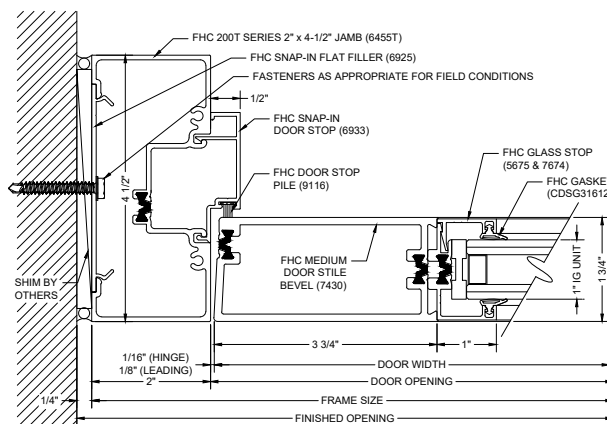
F13 DOOR JAMB @ WALL
