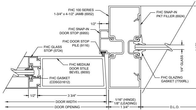
E2 DOOR & SIDELITE JAMB
