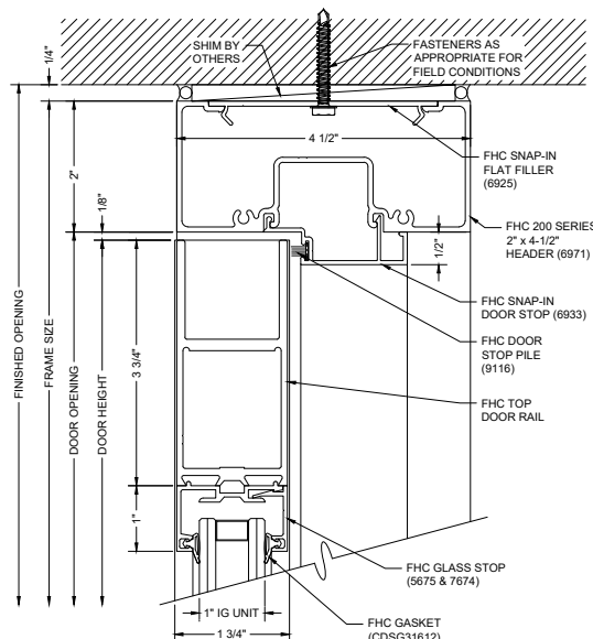
B3 DOOR HEADER
