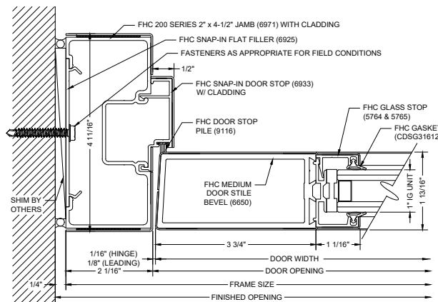
F11 DOOR JAMB @ WALL
