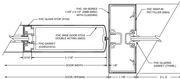
E20 DOOR & SIDELITE JAMB
