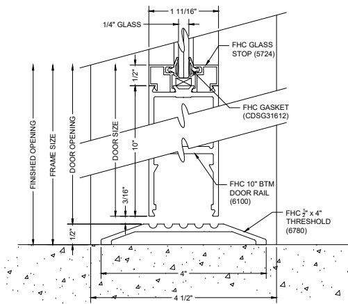
C6 BOTTOM OF DOOR
