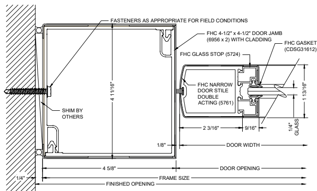
G30 DOOR JAMB @ WALL
