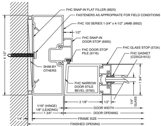
F1 DOOR JAMB @ WALL
