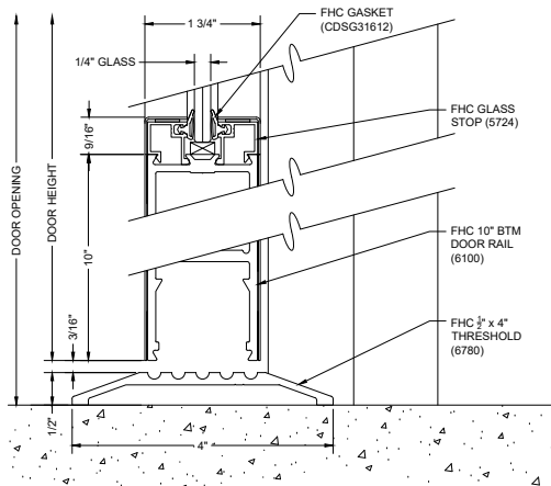
C2 BOTTOM OF DOOR
