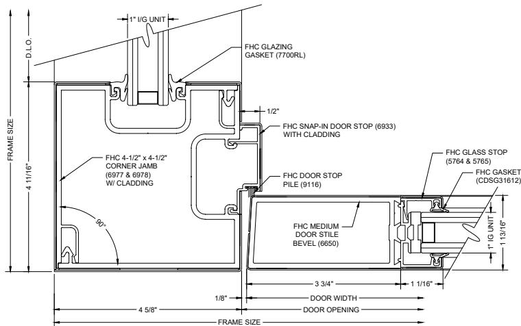
G11 90° CORNER DOOR JAMB
