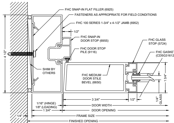
F2 DOOR JAMB @ WALL
