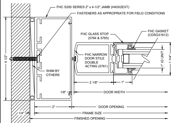
F21 DOOR JAMB @ WALL
