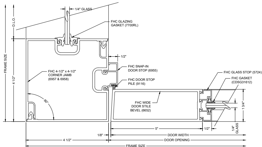
G3 90° CORNER DOOR JAMB
