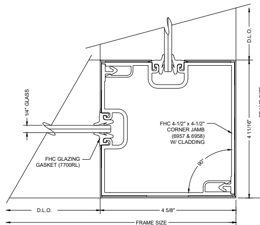
N4 90° CORNER JAMB
