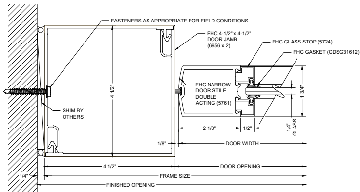
G27 DOOR JAMB @ WALL
