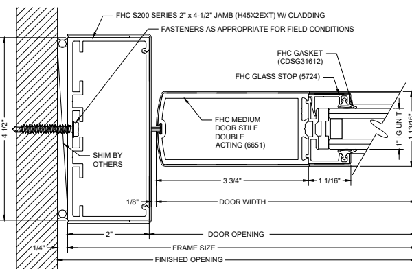
F25 DOOR JAMB @ WALL
